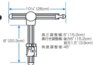
ヘッドレストスタンド
