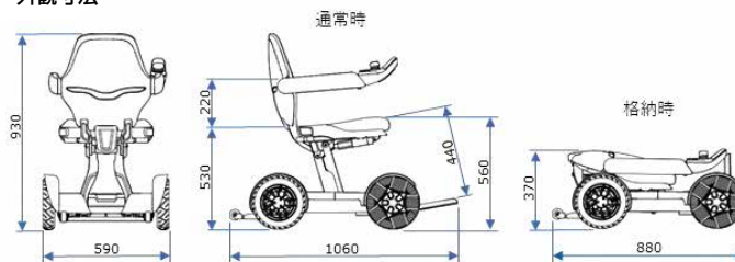
外観寸法
