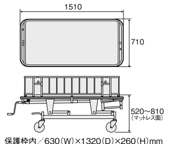
■寸法図(mm)
