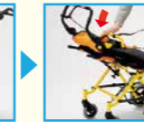
左側サイドプレートの「背もたれ誤動作防止装置」を解除してから、バックサポート角度変換ワイヤーを引いて、バックサポートを前方に倒します。
