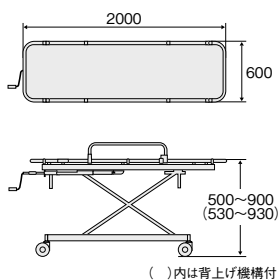
■寸法図(mm)
