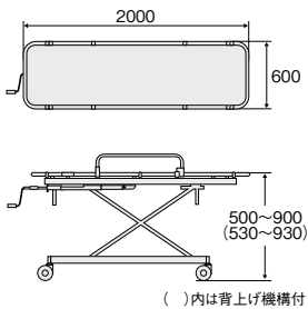
■寸法図(mm)
