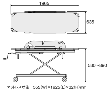
■寸法図(mm)
