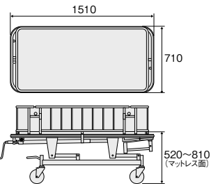
■寸法図(mm)
