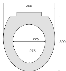
TY523・524座面寸法 単位:mm
