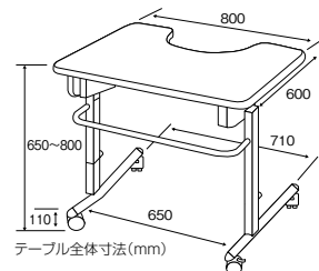
テーブル全体寸法(mm)
