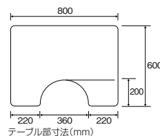
テーブル部寸法(mm)
