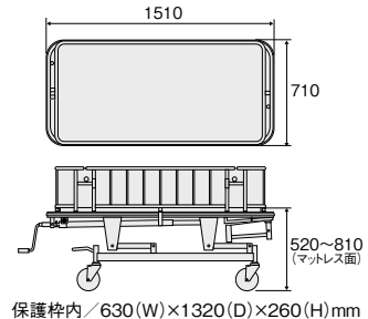
■寸法図(mm)
