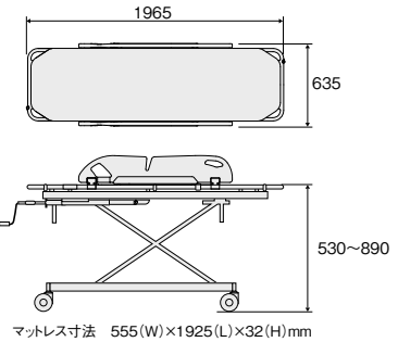
■寸法図(mm)
